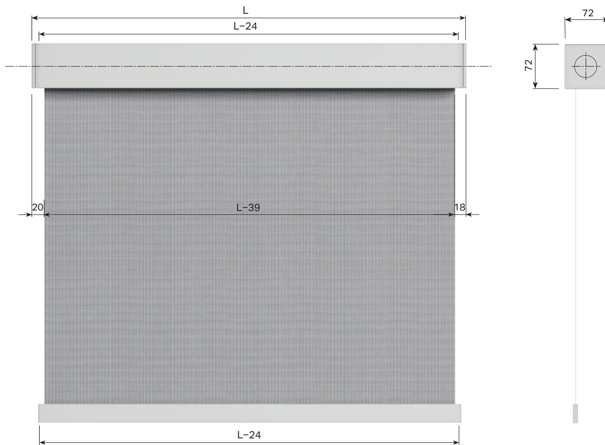
ROLLBOX 179
